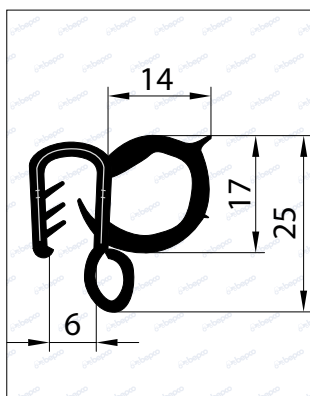
CLIPS BOUDIN AVEC PASSE FIL
