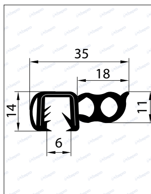
CLIPS BOUDIN DOUBLE SANS BUTYL
