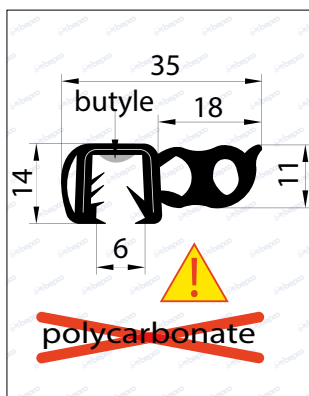
CLIPS BOUDIN DOUBLE AVEC BUTYL
